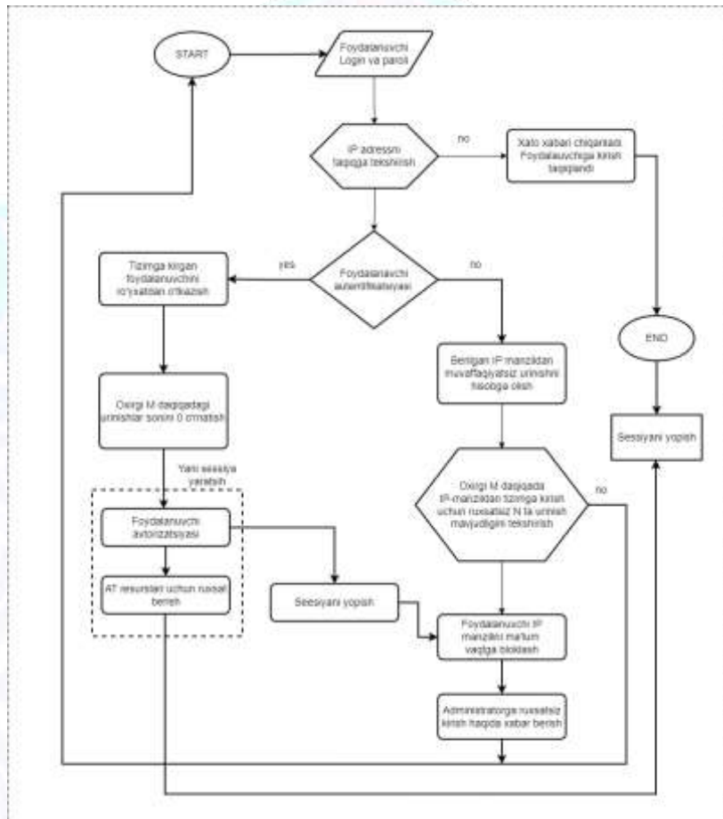
1-rasm. Vebga asoslangan axborot tizimlari autentifikatsiya jarayonida xavfsizlik algoritmi.
