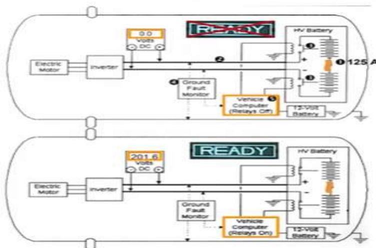
6-rasm. Gibrit avtomobilining xavfsizlik sistemasi
