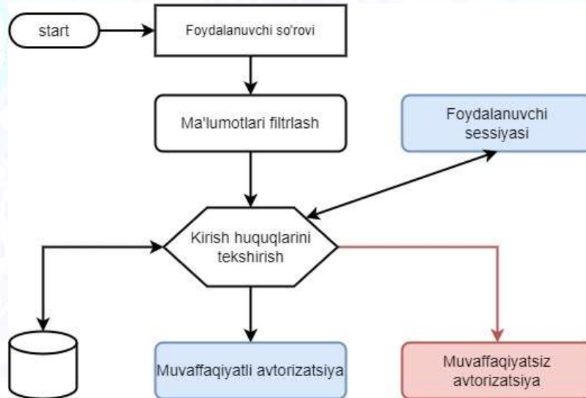
2-rasm. Vebga asoslangan axborot tizimlarida avtorizatsiyalash algoritmi.
