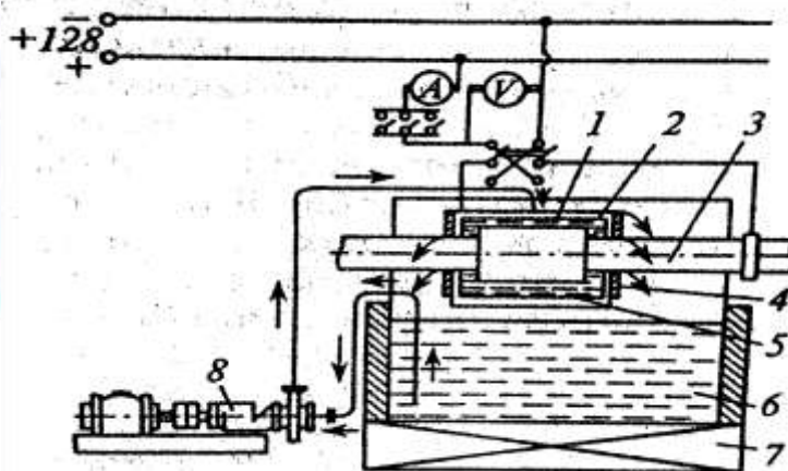
3 – rasm. Oqim bilan xromlash qurilmasining sxemasi:
