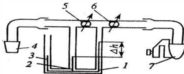
1 – rasm. KI – 4887 – 1 sarf oʻlchagichning sxemasi:
