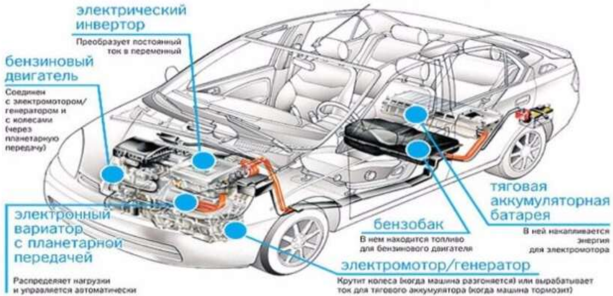
3-рasm. Гибрид avtomobilining uzal va agregatlari joylashuvi.
